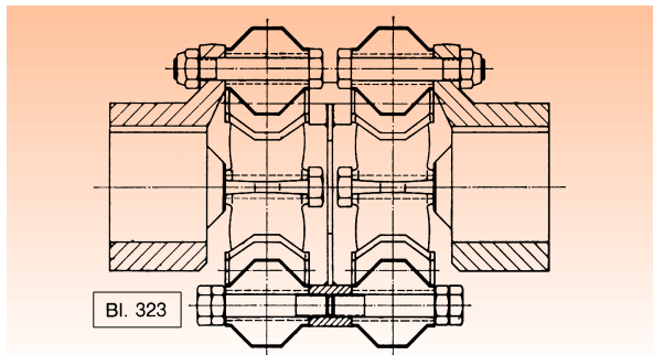
Kombinierte Hochelastische Doppelkupplung mit Zwischenflansch und normalen Flanschnaben (zur Verdoppelung der elastischen Werte für besondere Einbaufälle).
