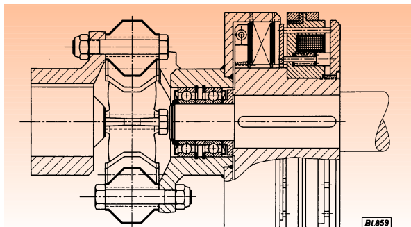
Hochelastische Kupplung als Nabenausführung kombiniert mit einer Elektromagnet-Lamellenkupplung.
